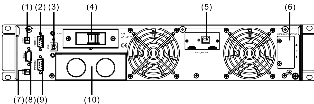
Задняя панель
