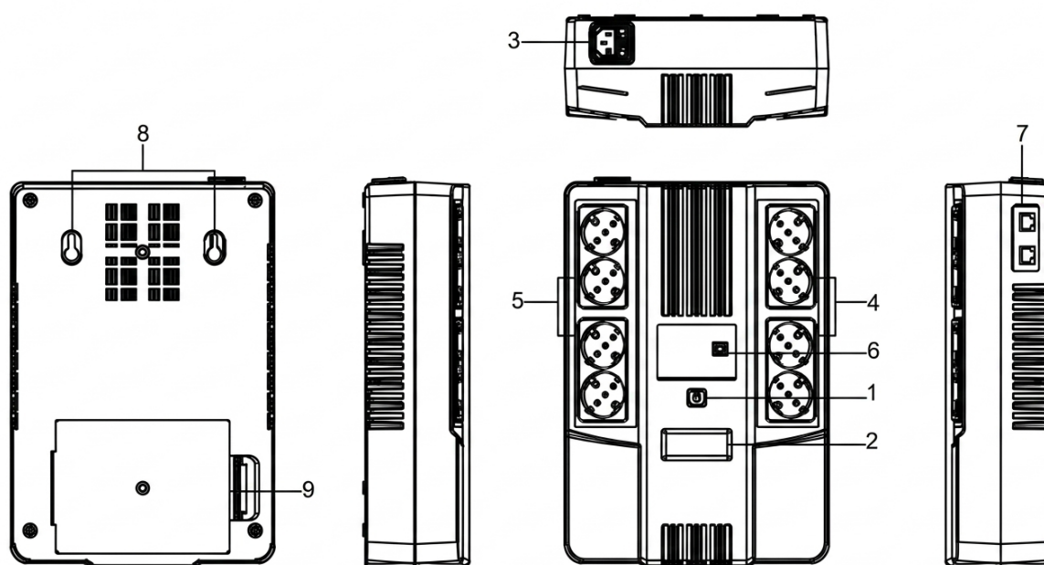
Рис.3. Задняя, передняя и боковые панели ИБП
